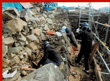
大洲城二の丸西曲輪石垣改修状況 （写真提供：大洲市教育委員会）
