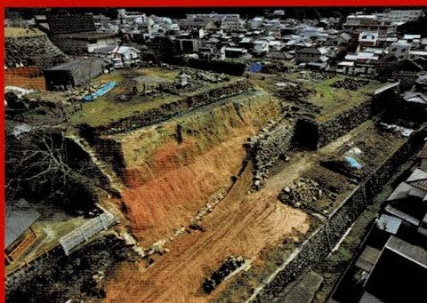
大洲城二の丸西曲輪石垣改修全景 （写真提供：大洲市教育委員会）
